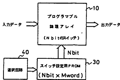
本発明の原理ブロック図 第1図
